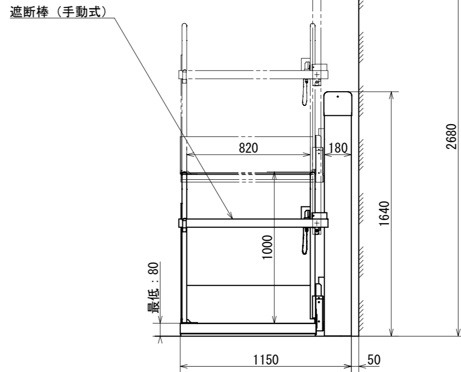
全体構造据付図 (DA-100Ad) 遮断棒付き
